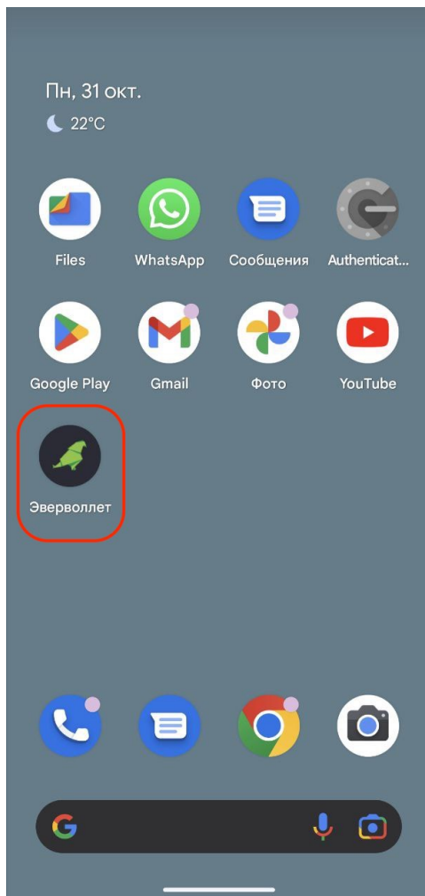
Рис. 7 Приложение установлено
